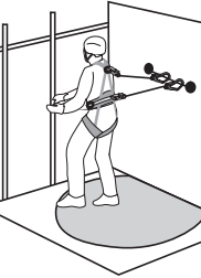
Рис. 13. Способ организации системы удержания
