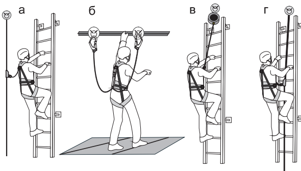
Рис. 13. Способ организации системы удержания
