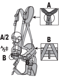
Рис. 3. Маркировка изделия
